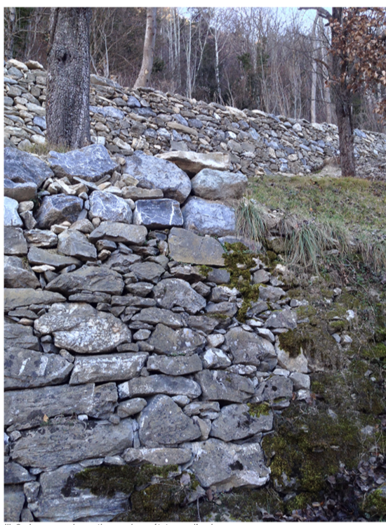
Ill. 2 : Les murs de soutien remis en état, vus d'en bas (photo : H. P. Kistler, Office fédéral des routes OFROU)
