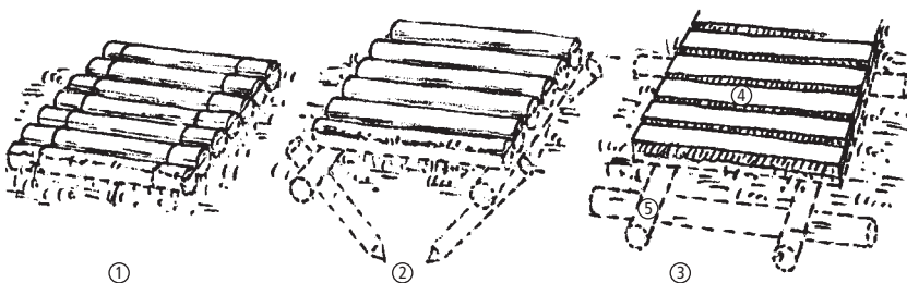
Struttura di semplici camminamenti a tavoloni o a tondelli: 1. tappeto di tondelli, 2. tappeto di tondelli con aumentata capacità di carico, 3. camminamento a tavoloni, 4. tavoloni, 5. tondelli (SAW/ASTRA 2001, 87).
